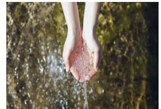
Juumaveden käsittelyratkaisut
